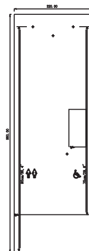
Plantilla de instalación
