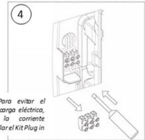
Desconectar los cables y quitar la regleta
