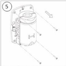
Desatornillar los tornillos de la pared (x4)
