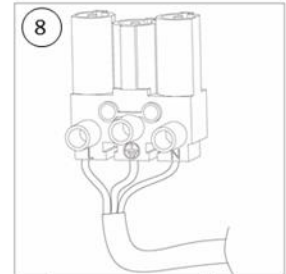
En la parte trasera del aparato, conectar los cables a la regleta siguiendo las letras marcadas en la regleta (N, L y Tierra)
