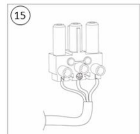
Conectar los cables al conector rápido siguiendo las letras marcadas (N, L y Tierra)
